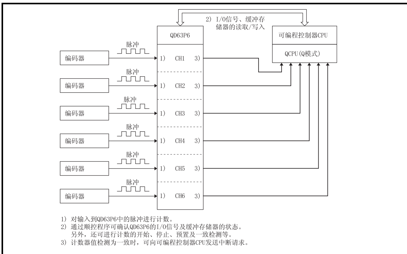
图 1.1 QD63P6 的动作概要
