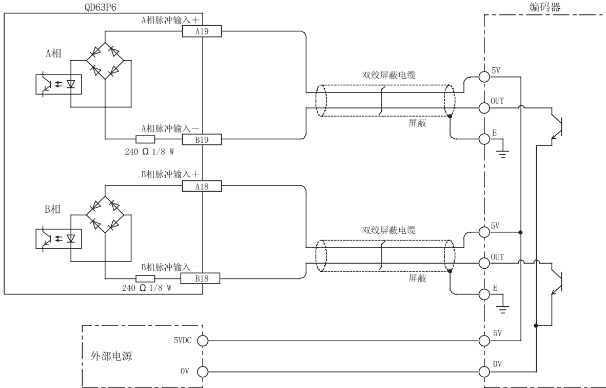
图 4.6 与编码器间 (DC5V 的情况下) 的接线示例
