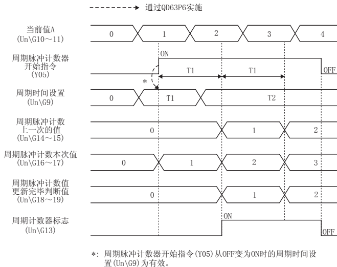
图 3.7 周期计数器标志 (Un\G13) 的时序图
