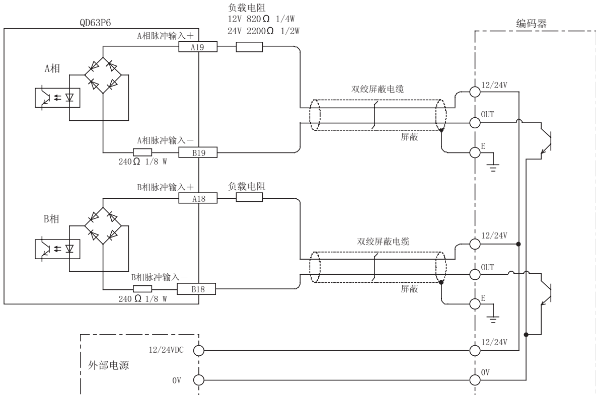
图 4.9 与编码器 (DC12/24V 的情况下) 的接线示例
