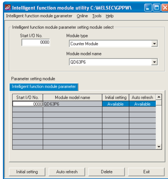
图 6.5 参数设置模块选择画面
