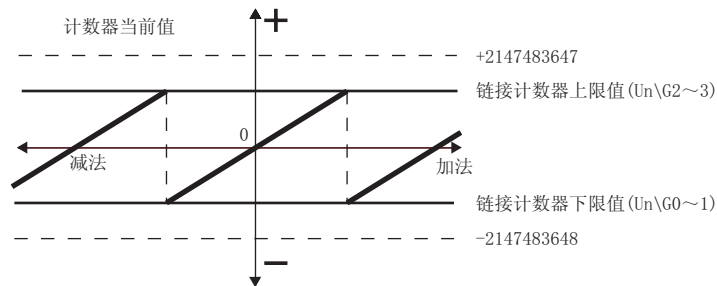
图 5.2 链接计数器的动作图
