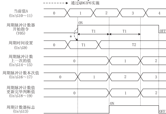
图 3.4 周期时间设置 (Un\G9) 的时序图
