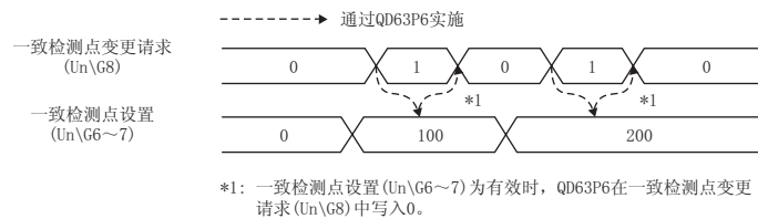
图 3.3 一致检测点设置 (Un\G6 ~ 7)、一致检测点变更请求 (Un\G8) 的时序图
