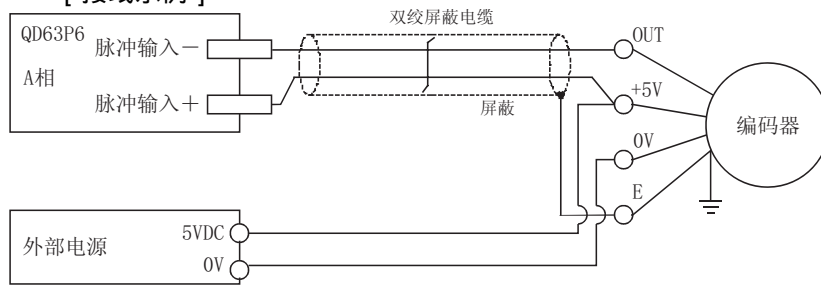
图 4.7 接线示例
