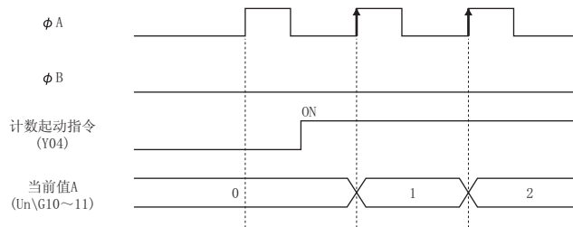
图 3.5 当前值 A(Un\G10 ~ 11) 的时序图
