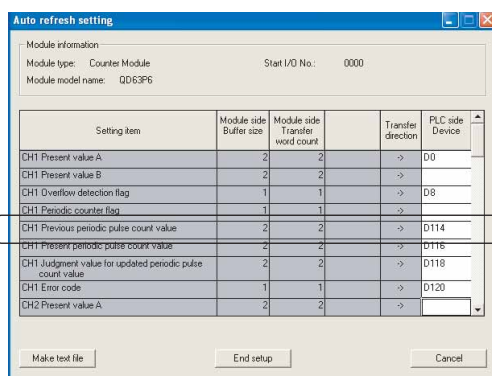
图 6.1 自动刷新设置的参数设置个数的计数方法
