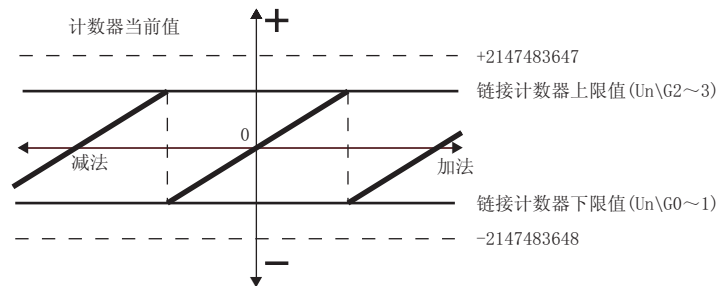
图 5.3 链接计数器的动作图 1
