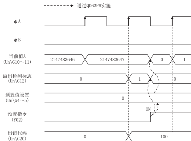
图 3.6 溢出检测标志 (Un\G12) 的时序图
