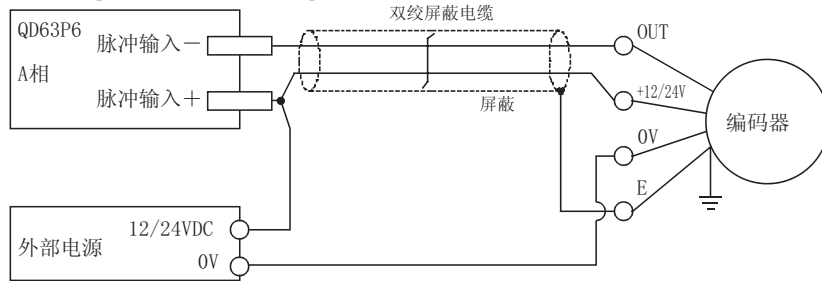
图 4.11 不良的接线示例
