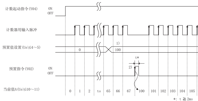
图 5.11 预置功能的动作示例
