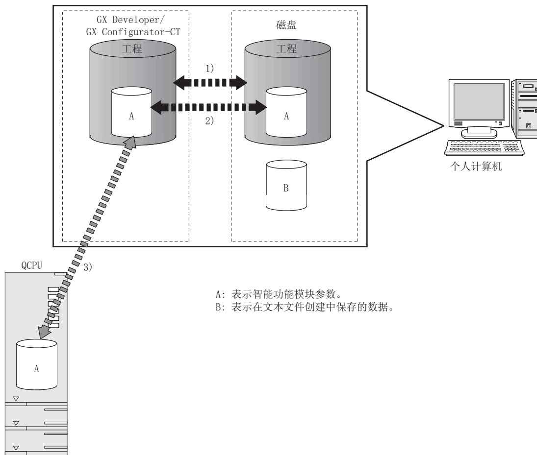
图 6.3 通过应用程序包创建的数据的相关图
