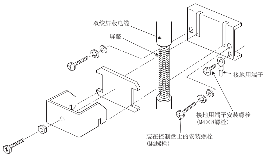
图 4.5 通过 AD75CK 进行的双绞屏蔽电缆的接地方法
