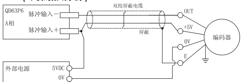
图 4.8 不良的接线示例
