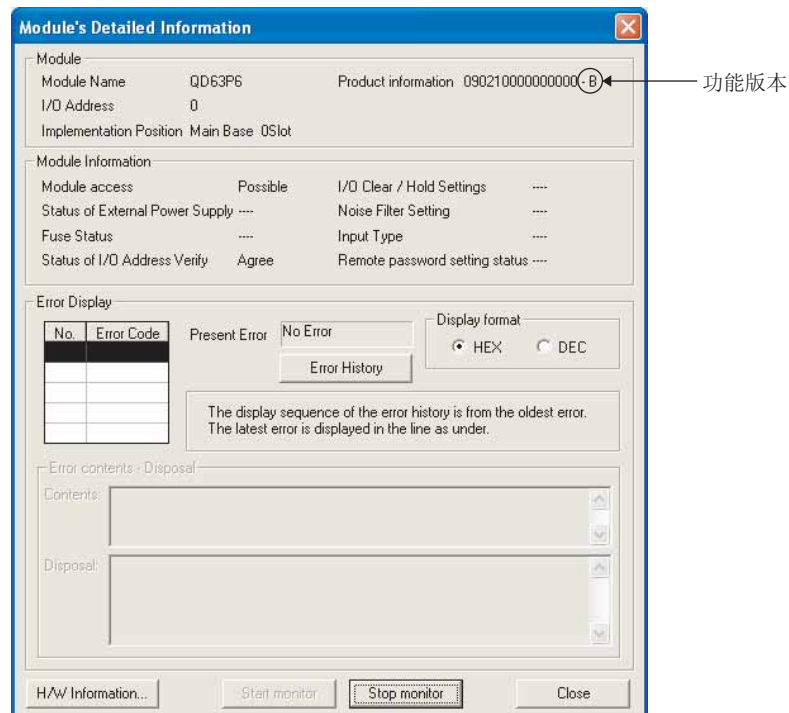
图 2.2 GX Developer 的模块详细信息对话框
