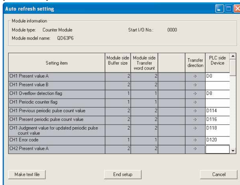
图 6.7 自动刷新设置画面
