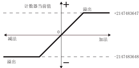
图 5.1 线性计数器的动作图
