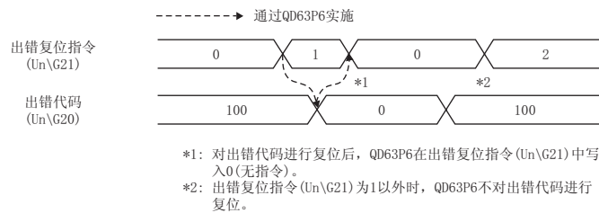
图 3.8 出错复位指令 (Un\G21) 的时序图
