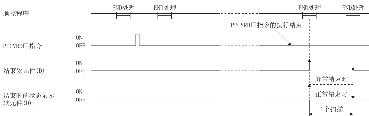
附图 2 PPCVRD 指令的时序图
