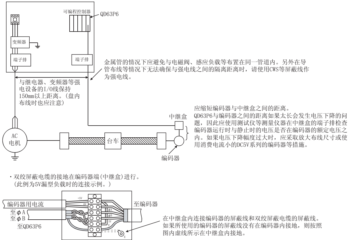
图 4.3 噪声解决方案接线示例
