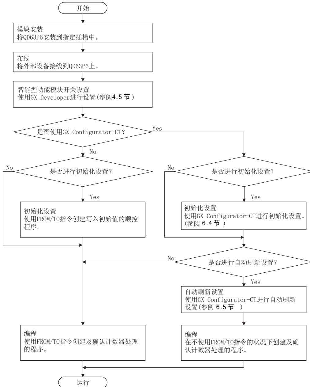
图 4.1 投运前的步骤
