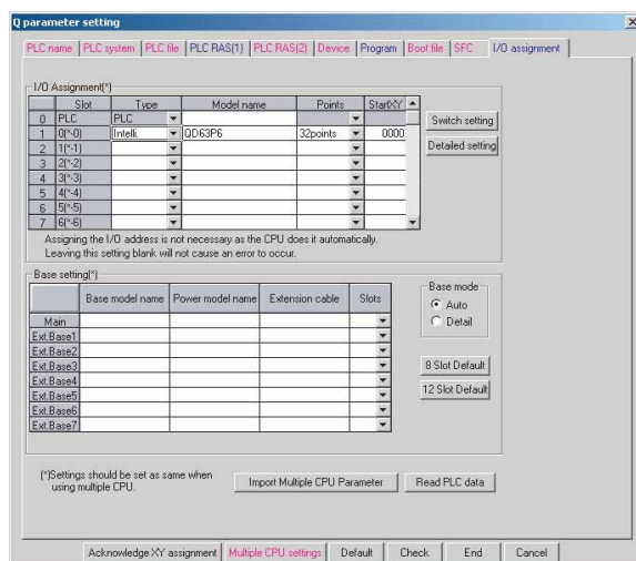
图 4.14 I/O 分配设置示例
