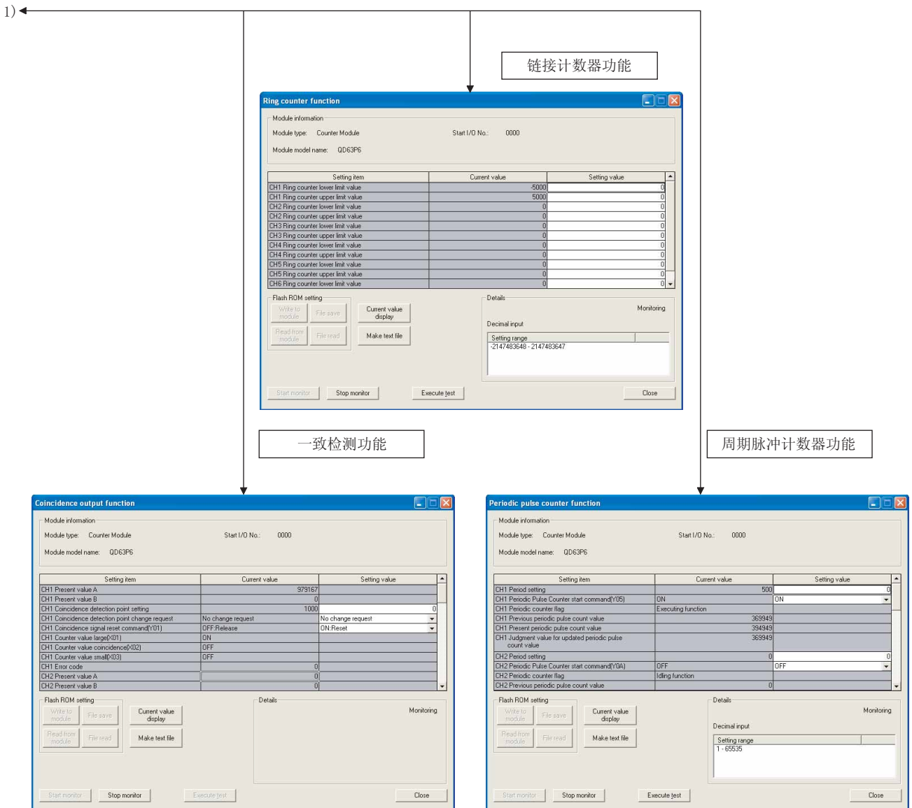
图 6.8 监视 / 测试画面 (续)
