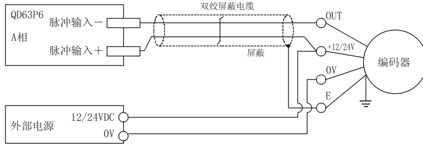
图 4.10 接线示例
