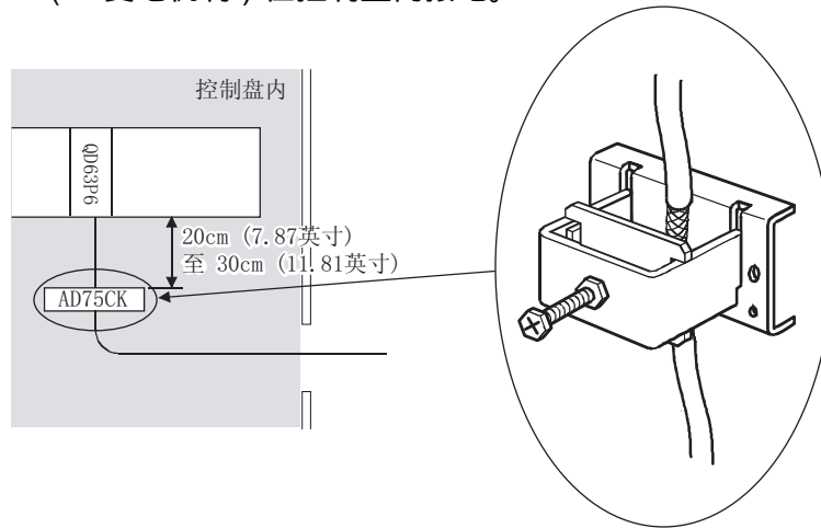
图 4.4 AD75CK 型电缆夹
