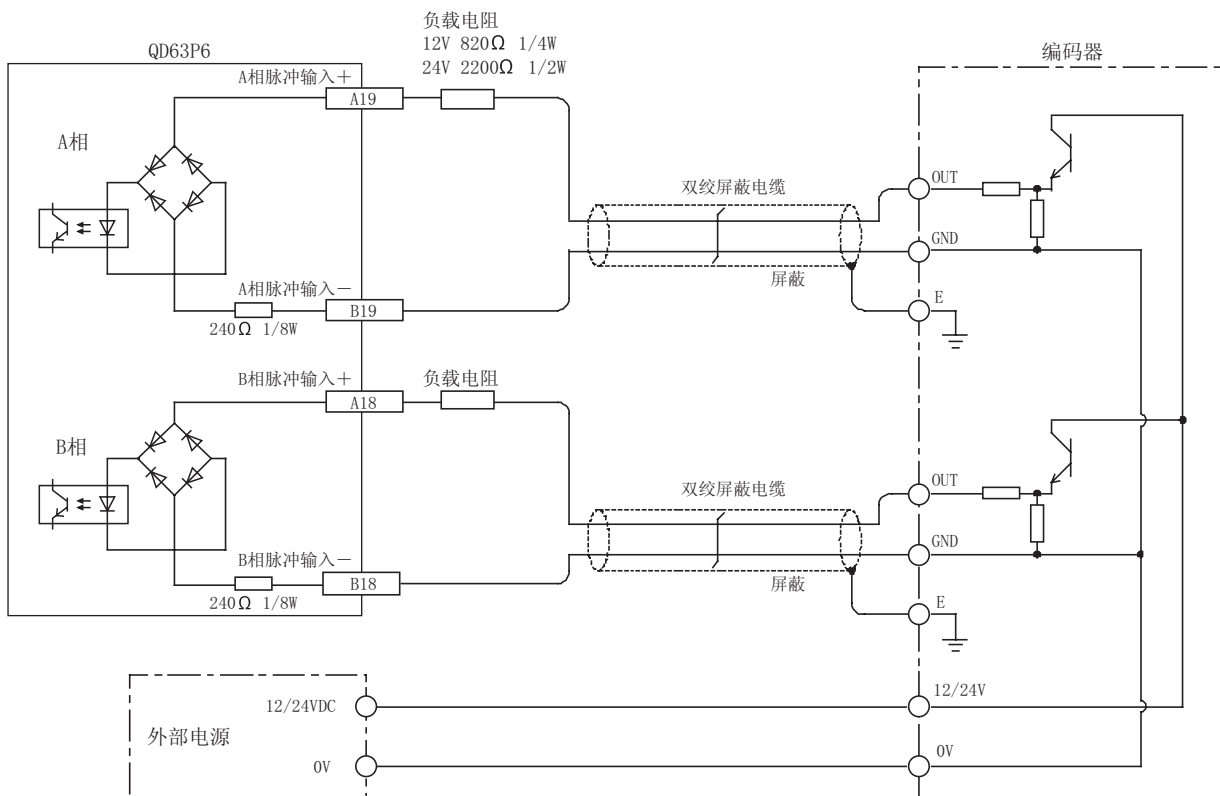
图 4.13 与编码器 (DC12/24V 的情况下) 的接线示例
