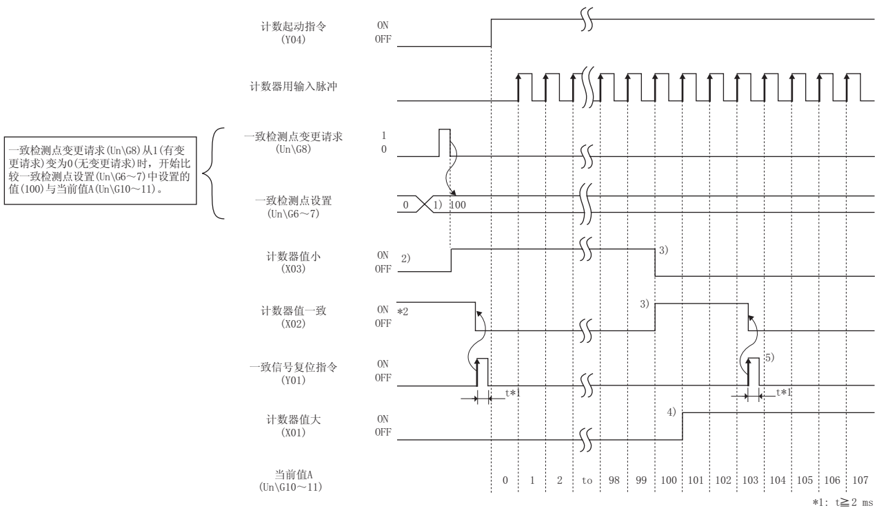
图 5.8 一致检测功能的动作示例
