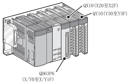
图 7.1 系统配置
