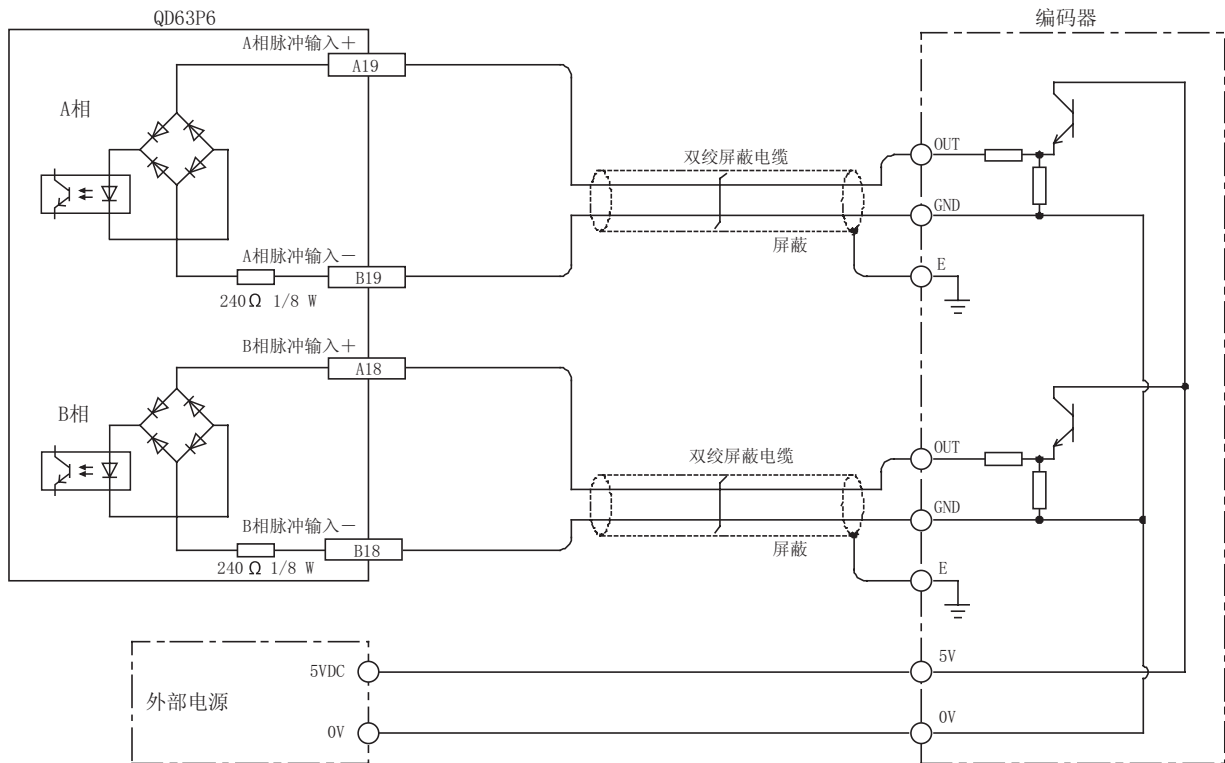
图 4.12 与编码器 (DC5V 的情况下) 的接线示例
