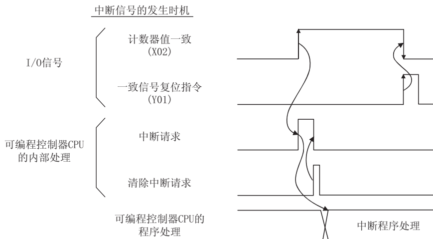
图 5.9 中断信号发生的时机
