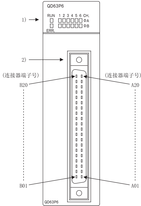
图 4.2 QD63P6 的外观
