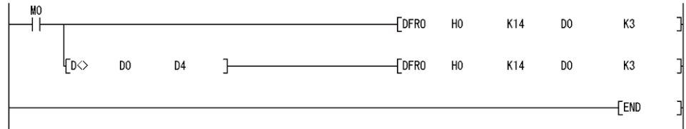
图 5.13 : 周期脉冲计数值读取程序示例
