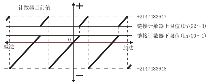
图 5.5 链接计数器的动作图 2
