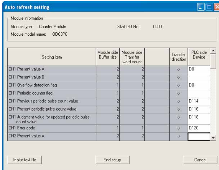
图 7.3 自动刷新设置画面
