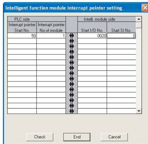
图 7.5 智能功能模块中断指针设置
