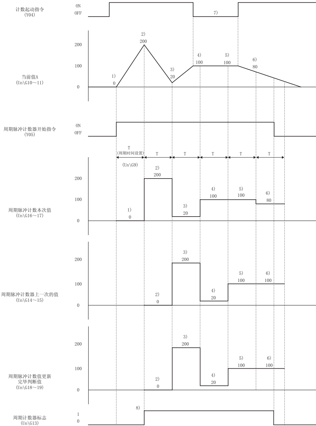
图 5.12 周期脉冲计数器功能的动作示例
