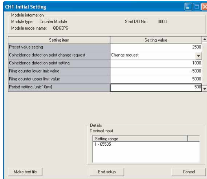
图 7.2 初始化设置画面
