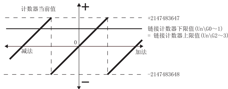
图 5.7 链接计数器的动作图 3
