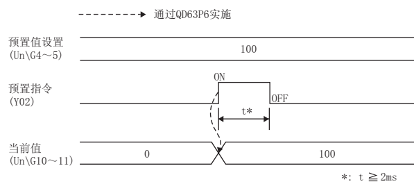
图 3.2 预置值设置 (Un\G4 ~ 5) 的时序图
