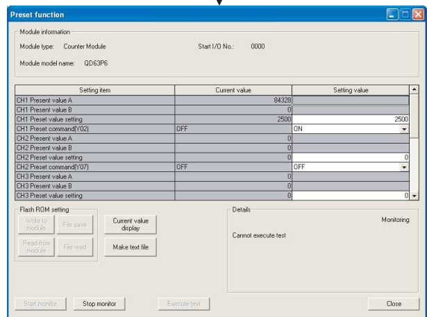
图 6.8 监视 / 测试画面
