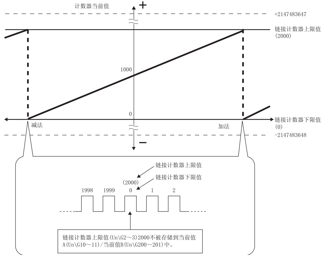
图 5.4 链接计数器的动作示例 1
