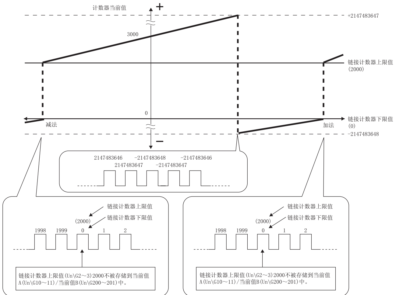
图 5.6 链接计数器的动作示例 2
