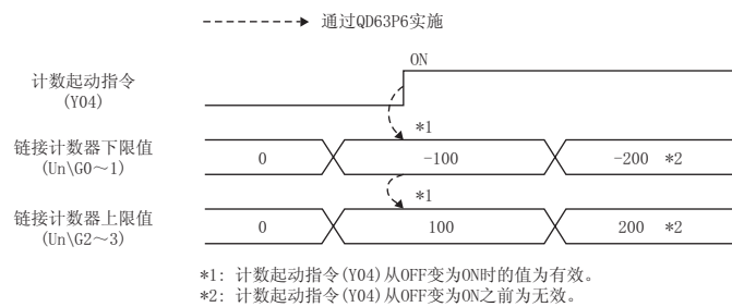
图 3.1 链接计数器下限值 (Un\G0 ~ 1)、链接计数器上限值 (Un\G2 ~ 3) 的时序图
