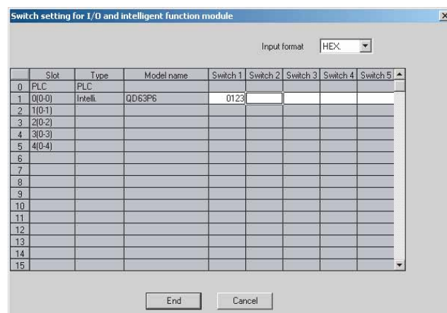
图 4.15 I/O 模块、智能功能模块开关设置画面
